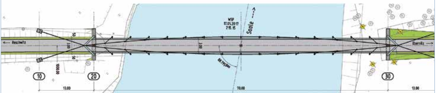
Radwegebrücke - Draufsicht
